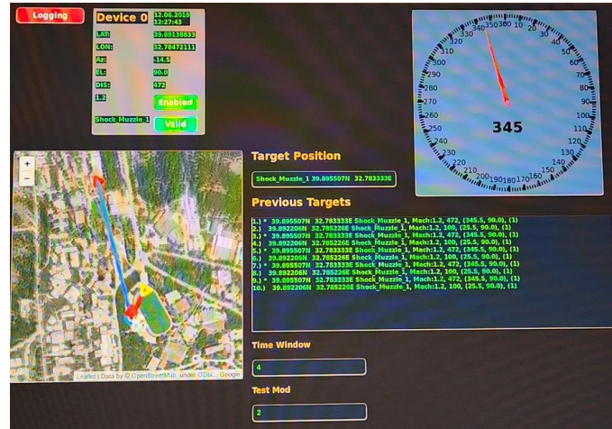
Kullanıcı Ekranı
